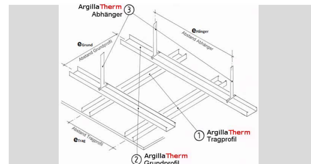
3. Die Metalldecken-Abhängung in Leichtbauweise, freitragend oder mit Deckenabhänger
